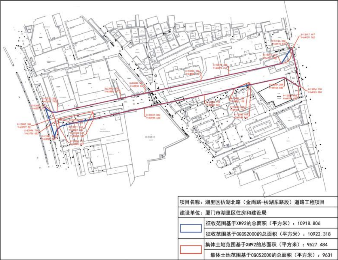
湖里区枋湖北路（金尚路-枋湖东路段）道路工程项目征收范围图
